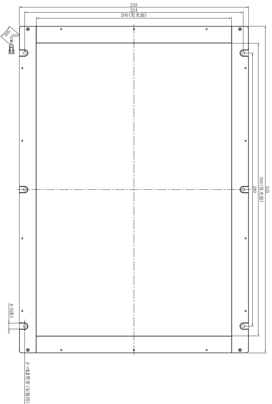
产品安装尺寸图
