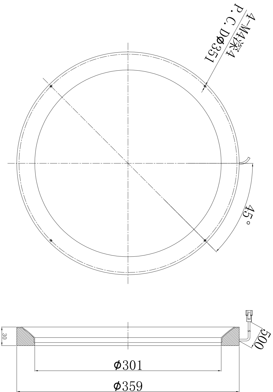
产品安装尺寸图
