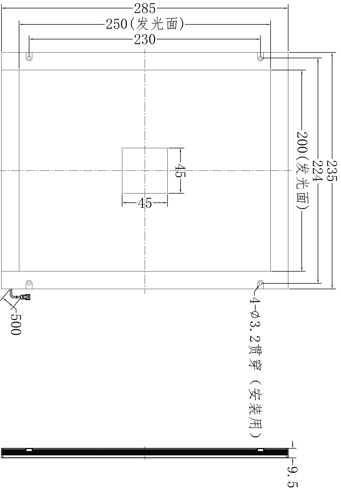
产品安装尺寸图
